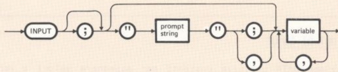
Figura 5-7 Istruzione INPUT
